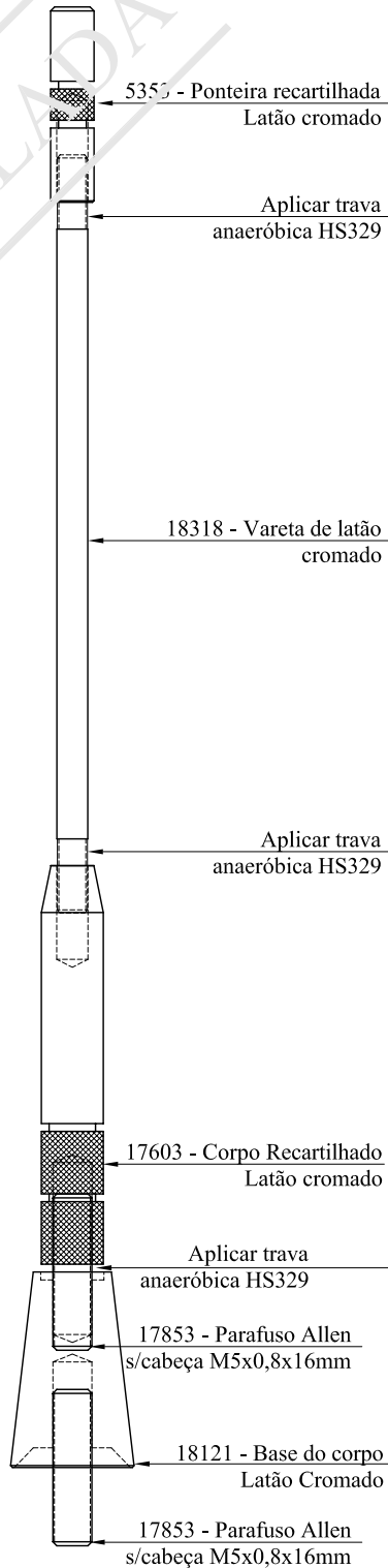
VISTA EXPLODIDA 4096 - Subconjunto Mini Haste Recartilhada Vareta Cromada
