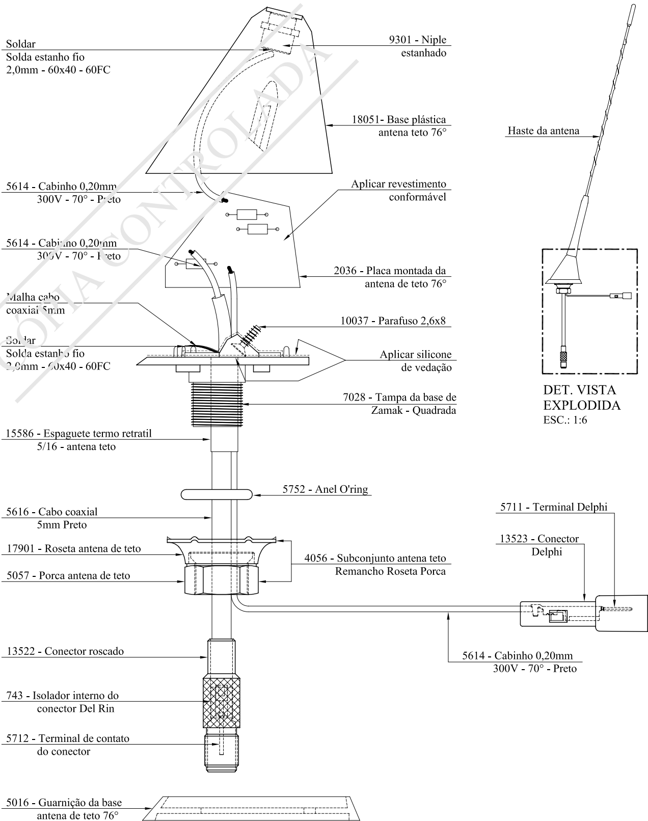
VISTA EXPLODIDA ESC.: 1:1
