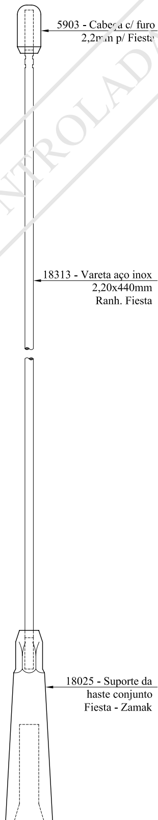
VISTA EXPLODIDA 3917 - Subconjunto haste Fiesta preta ESC.: 1:1
