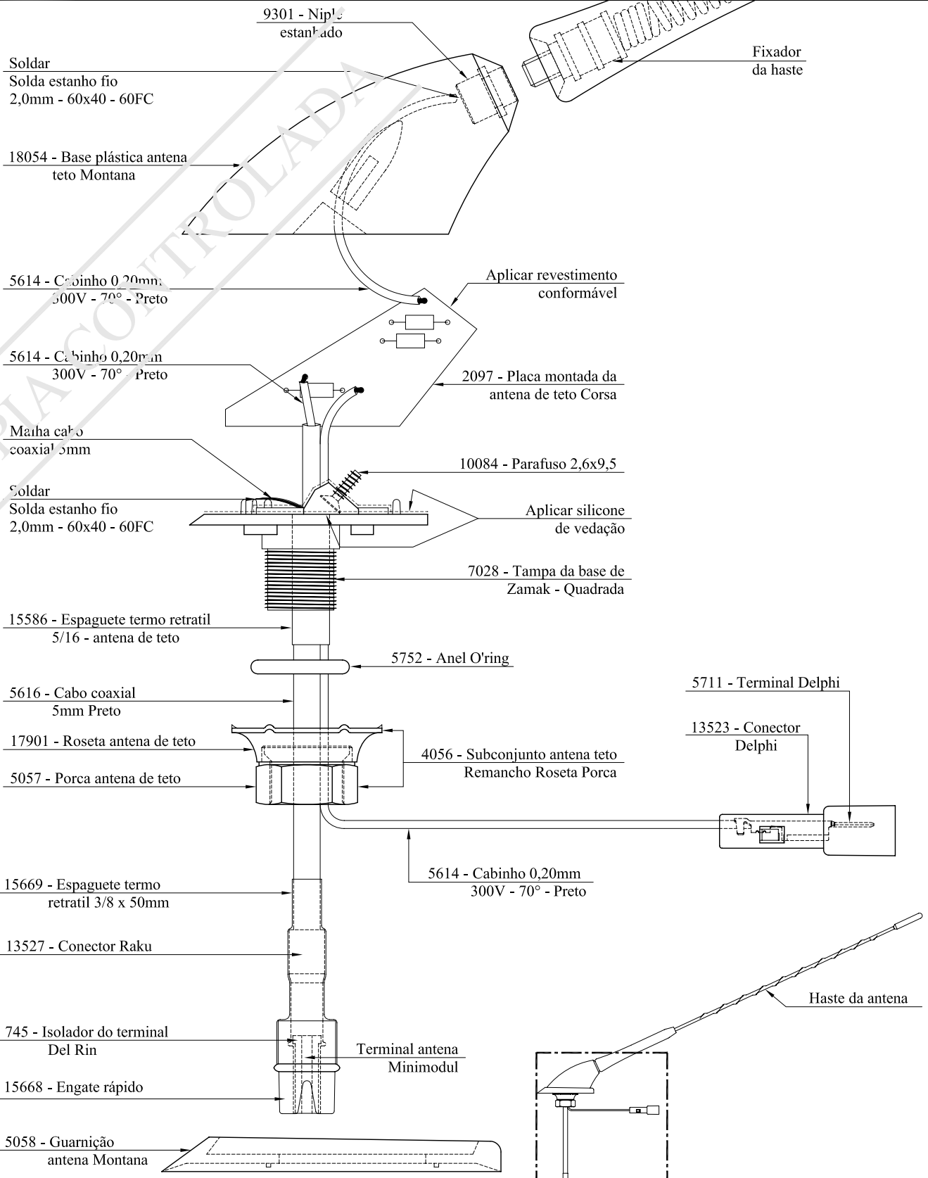
DET. VISTA EXPLODIDA ESC.: 1:6
