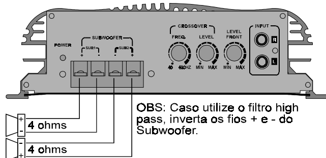
SUBWOOFERS (CAIXA OU TAMPÃO)
