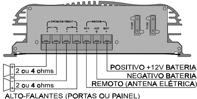
ALTO-FALANTES (PORTAS OU PAINEL)
